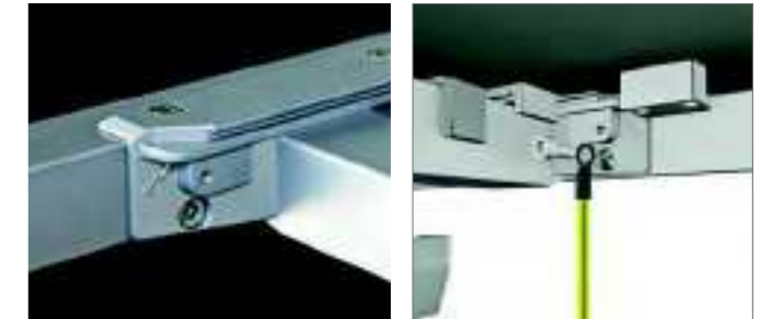
Punto de conexión a toma de tierra Earth wire point Point de connexion de prise en terre Anschlusspunkt für die Schutzleitung zur Erdung
