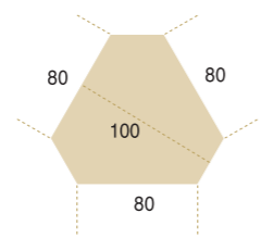
Ángulo 3 salidas Ángulo / Desk Link / Angle
